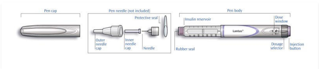
SoloStar Enjeksiyon Kalemi Şematik Çizimi
